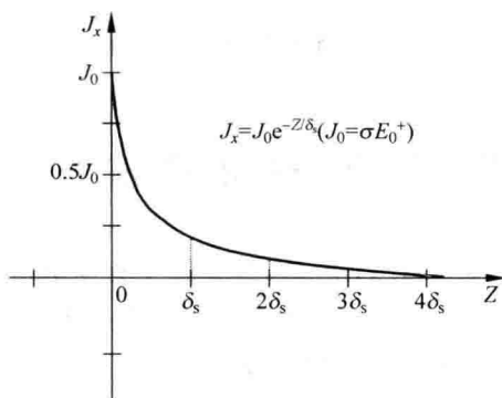
图 1.8 趋肤效应曲线图
