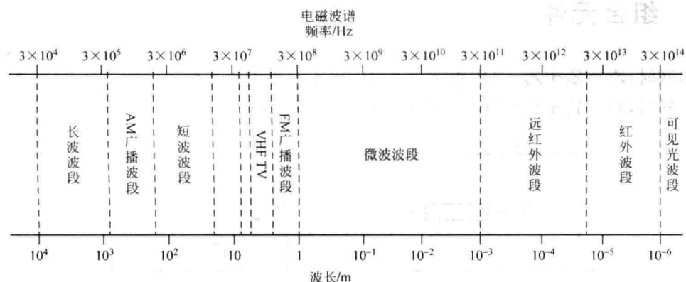
图 1.1 电磁微波频谱
