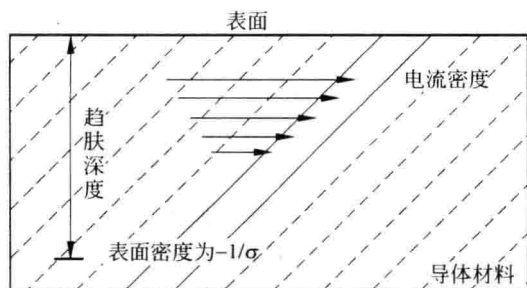
图 1.7 趋肤效应
