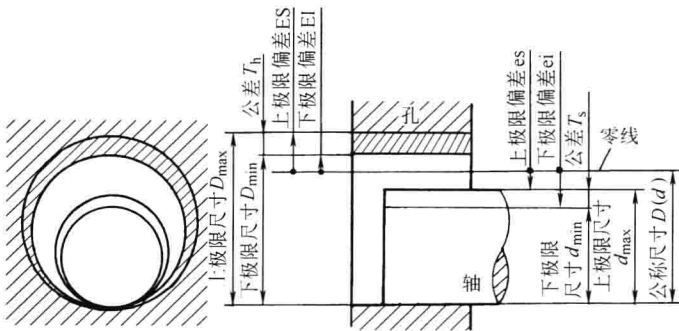
图 2-2 极限与配合示意图
