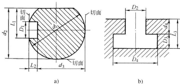
图 2-1 孔与轴的示例
