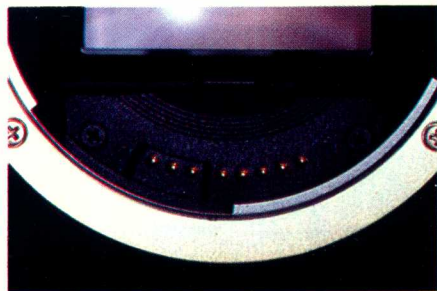
鏡身直驅自動對焦 鏡頭與機身耦合處八個電子觸點，傳遞訊號指令鏡頭內置馬達對焦，扭力充沛，快速寧靜。
