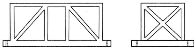
图 1-2 钢筋混凝土剪力撑结构设计示意图
