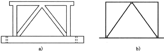
图 1-1 钢筋混凝土剪力撑结构锥形示意图 a) 形状示意图;b) 结构计算简图
