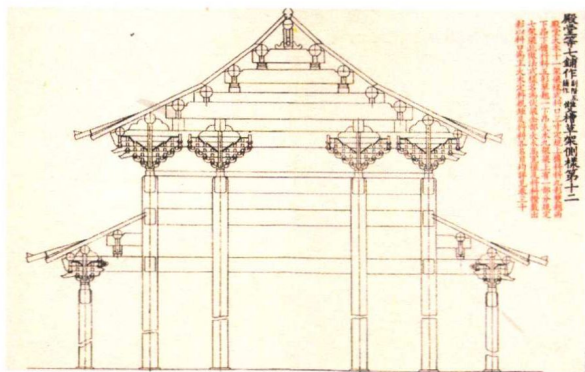
仿宋本《营造法式》（部分）
