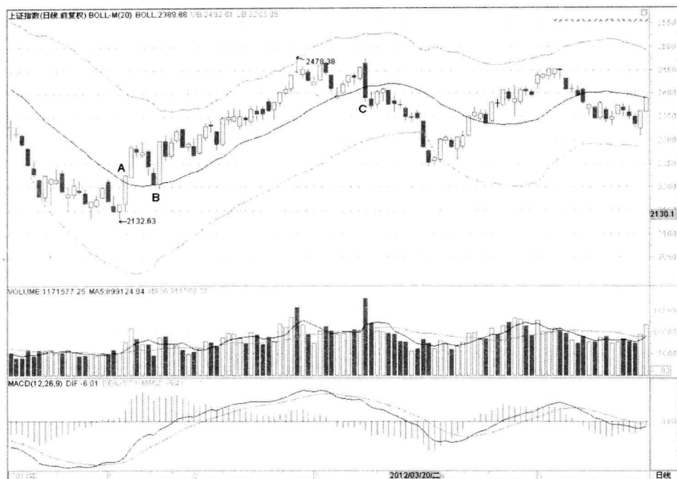
图 1-8 上证指数 (II) 999999
