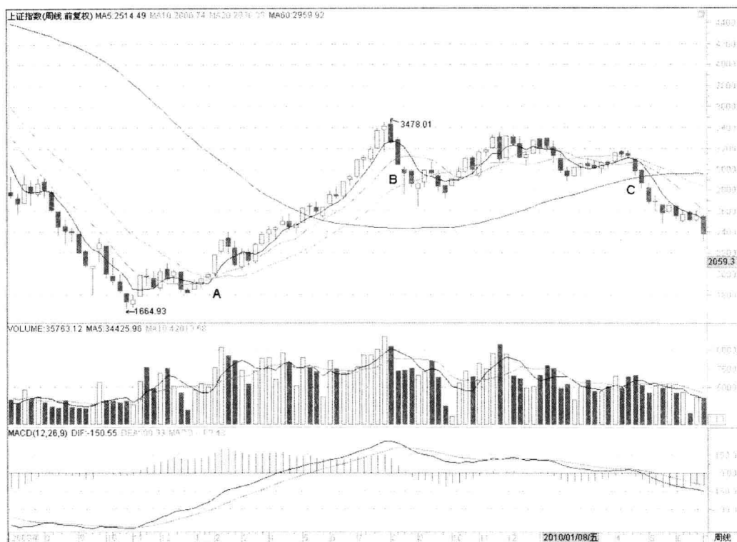
图 1-7 上证指数 (I) 999999
