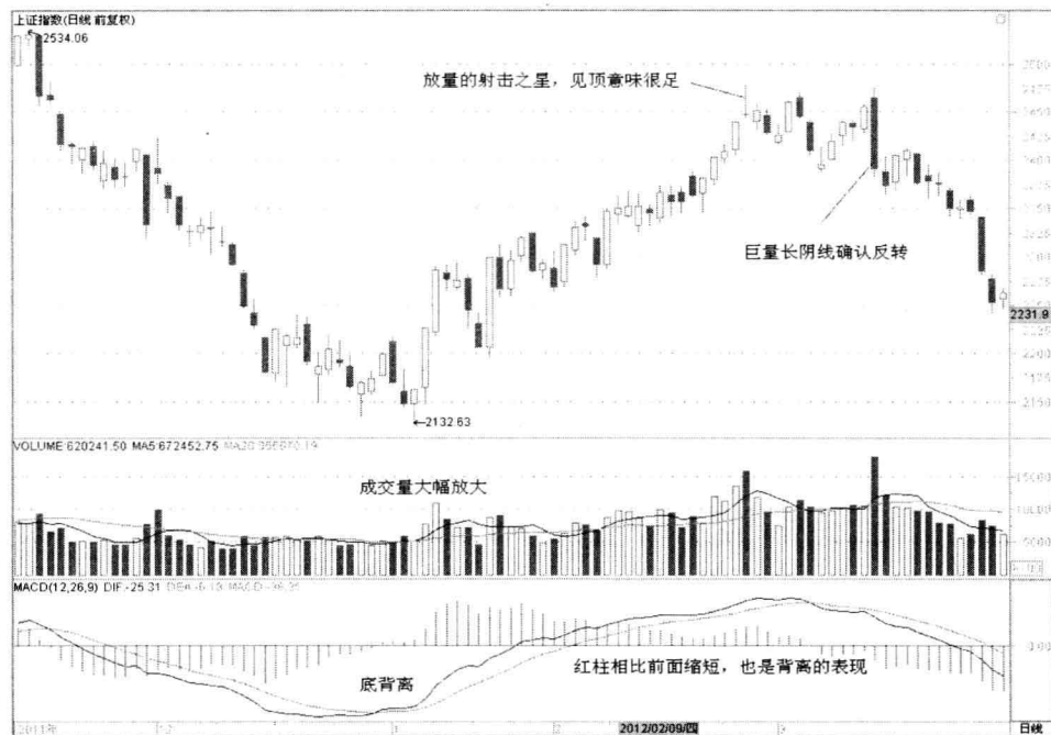
图 1-9 上证指数 (III) 999999
