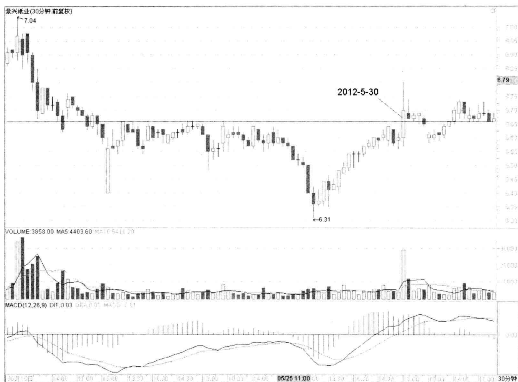
图 1-5 景兴纸业（I） 002067
