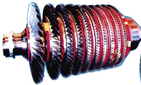
转子
