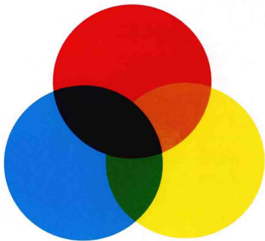
图1-2 色彩三原色
