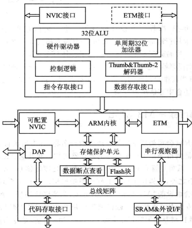
图 1.1.1 Cortex-M3 处理器内部架构一览
