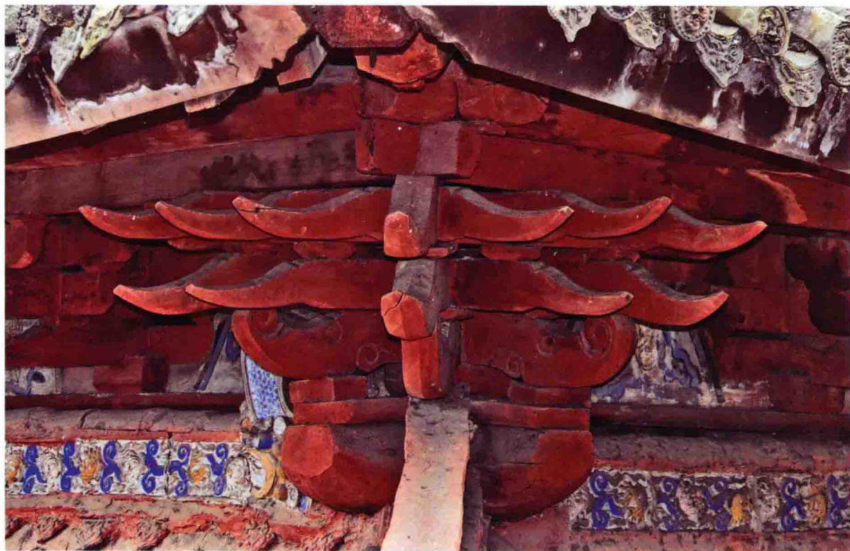
岱岳殿转角铺作（上檐）
