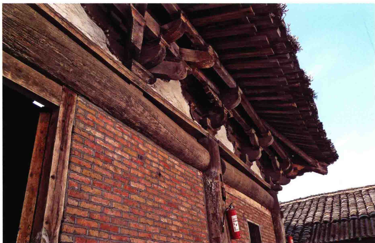
正立面局部
