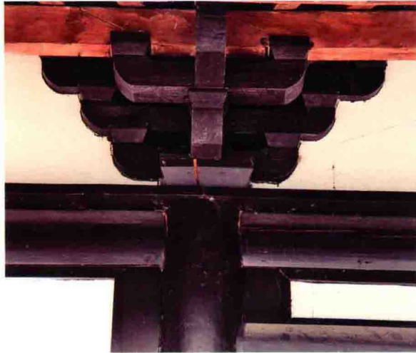
柱头铺作
