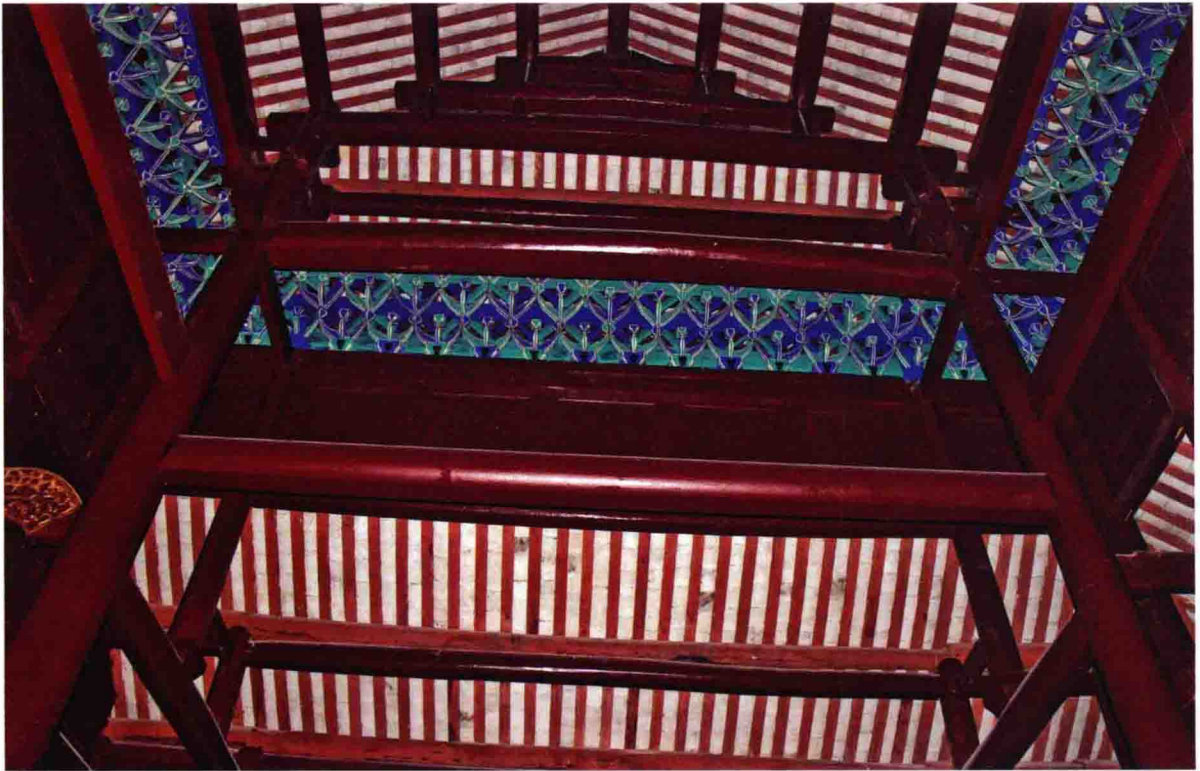
正殿梁架结构
