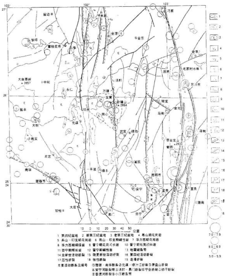
滇中地区地震构造图
