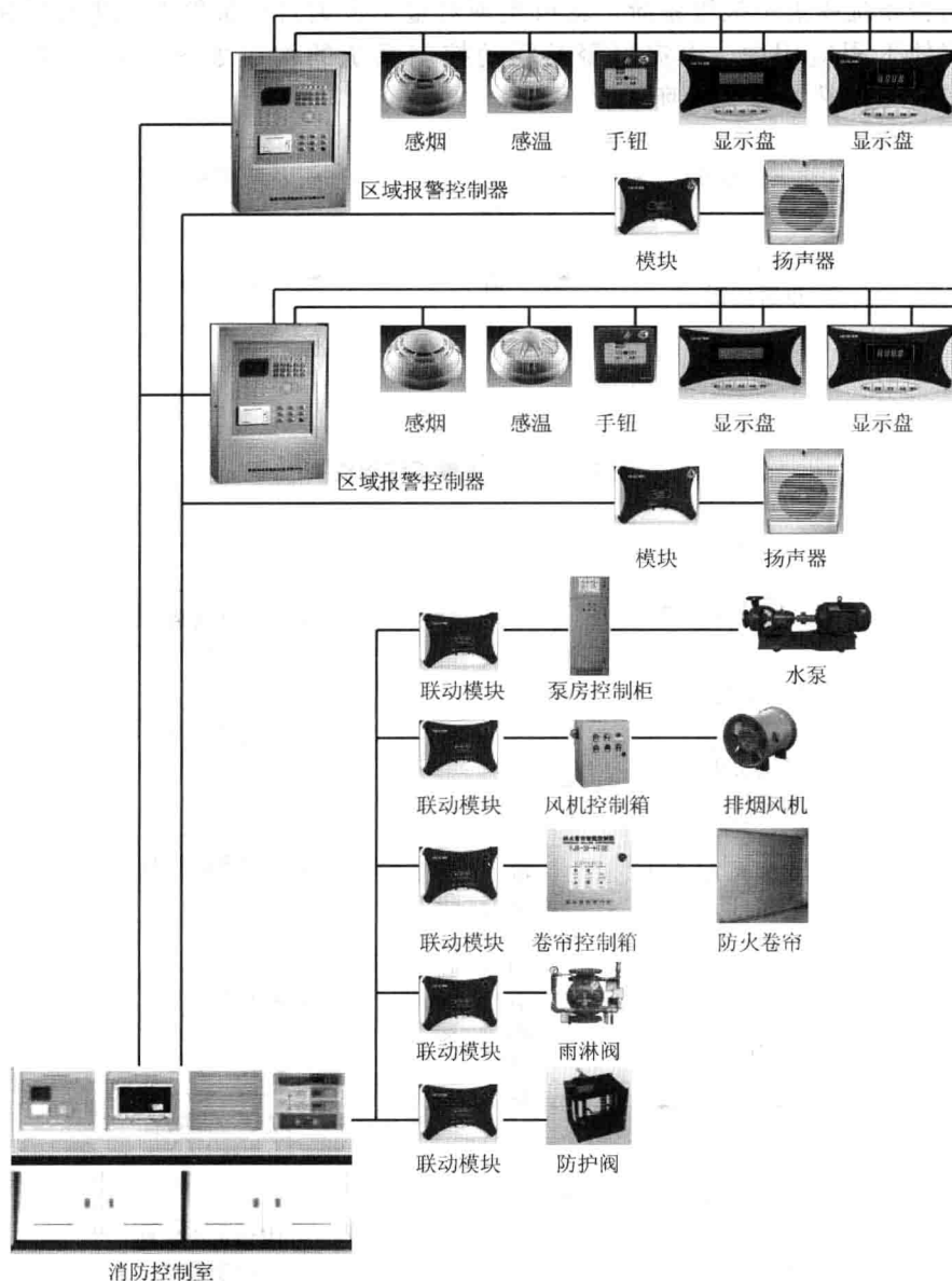
图 1-2-3 控制中心报警系统结构形式简图
