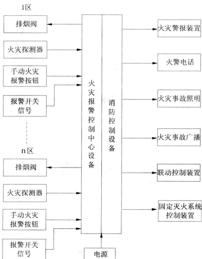
图 1-2-5a 控制中心报警系统组成
