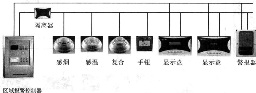
图 1-2-1 区域报警系统结构形式简图
