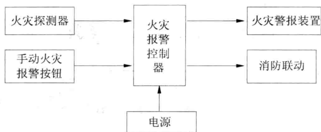
图 1-2-4 报警系统组成
