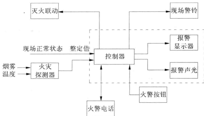
图 1-2-6 火灾自动报警系统原理框图
