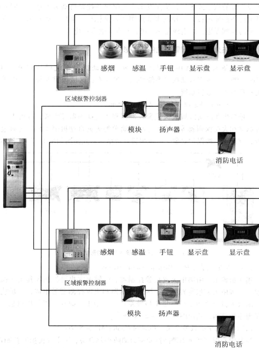
图 1-2-2 集中报警系统结构形式简图
