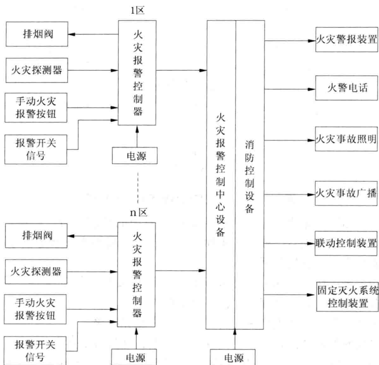
图 1-2-5b 控制中心报警系统组成
