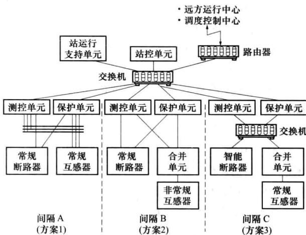
图 GYBD00101003-1 过程层常规设备接入方案
