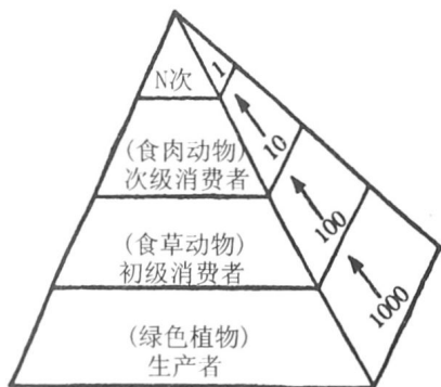
图 1-6 能量流动的生态金字塔 (来源:文献[6])
