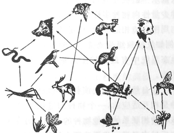
图 1-7 一种简化的温带针阔叶混交林中的食物网 (来源:文献[2])
