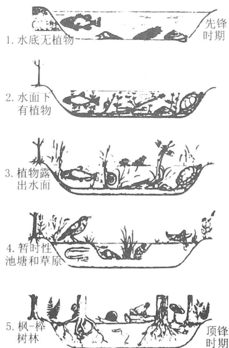
图 1-8 从池塘到森林的演替
