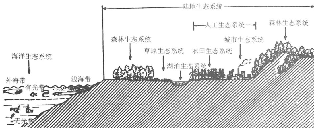
图 1-2 地球上生态系统的类型
