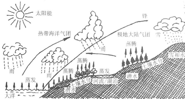
图1-5 地球生态系统的水循环
