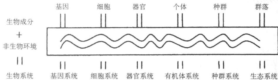
图 1-1 生态学研究的不同层次对象
