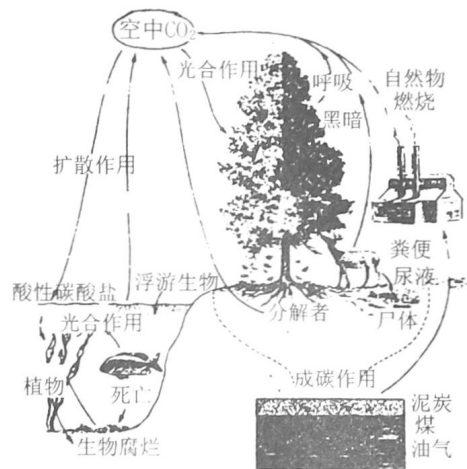
图1-4 地球生态系统中的碳循环
