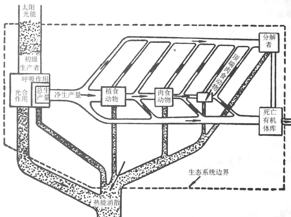
图 1-3 生态系统中的能量逐级流动
