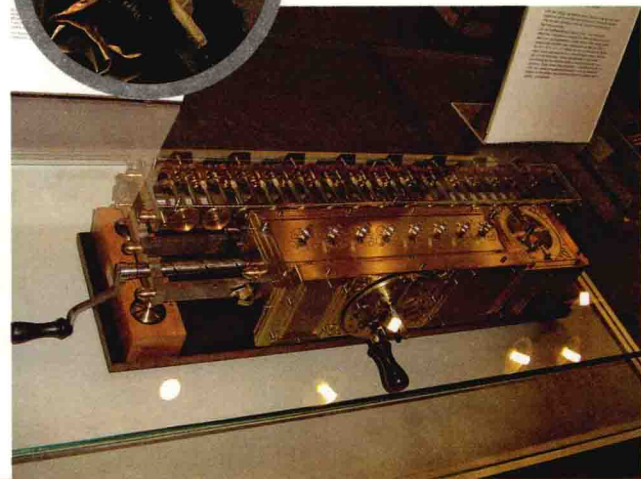
莱布尼茨发明的计算器复制品
