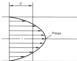
图 1-4 液体在管路内的速度分布
