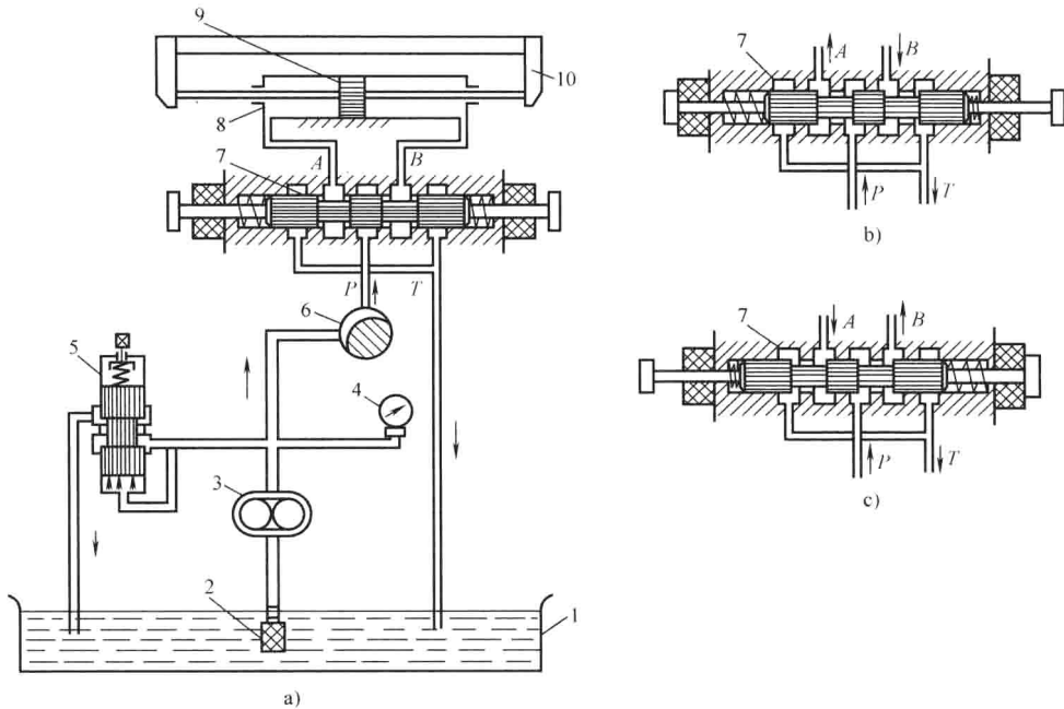
图 1-2 简化了的机床工作台的液压传动系统图
