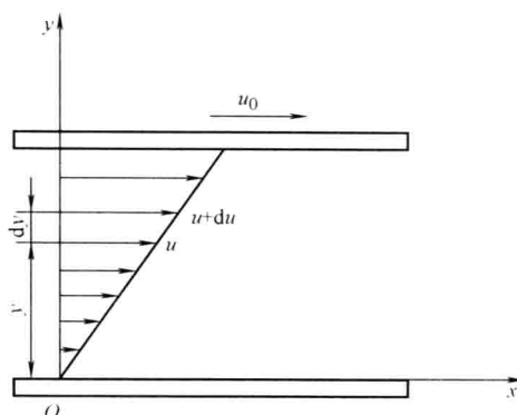
图 1-5 液体粘性示意图
