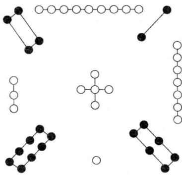
洛书
