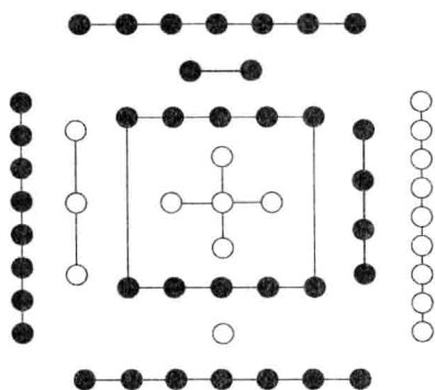
河图
