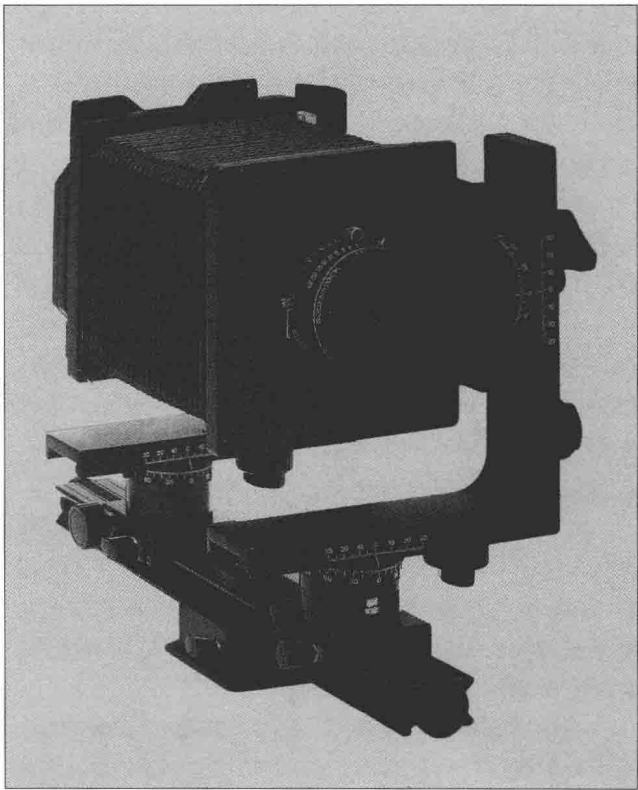
图2-1 4 \times 5 英寸单轨相机
