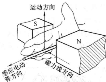
图 1-5 右手定则
