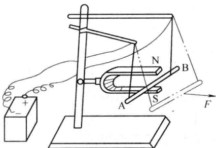
图 1-4 直导体切割磁力线运动
