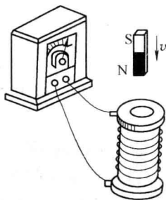
图 1-6 线圈中的感应电动势
