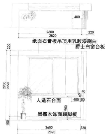
餐厅C立面图
