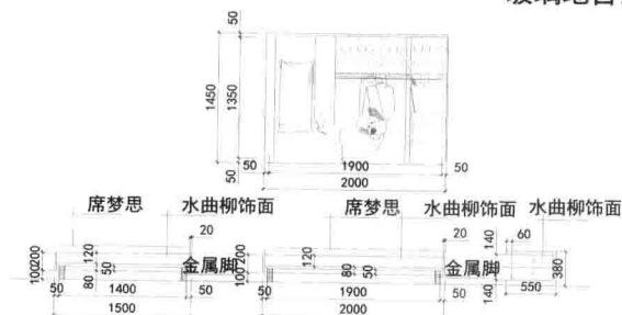
女孩房床、床头柜立面图
