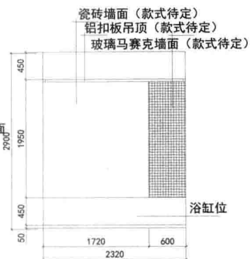
主卧室卫生间C立面图
