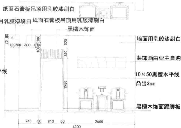
书房D立面图
