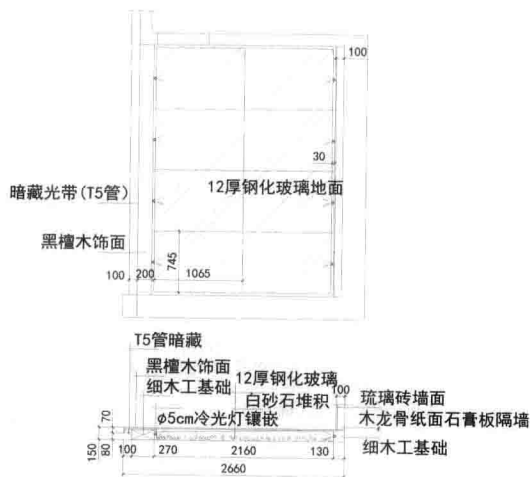
玻璃地台详图
