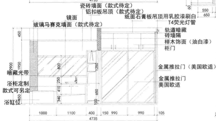
主卧室卫生间衣帽间D立面图
