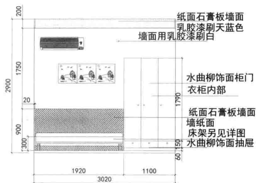
女孩房B立面图
