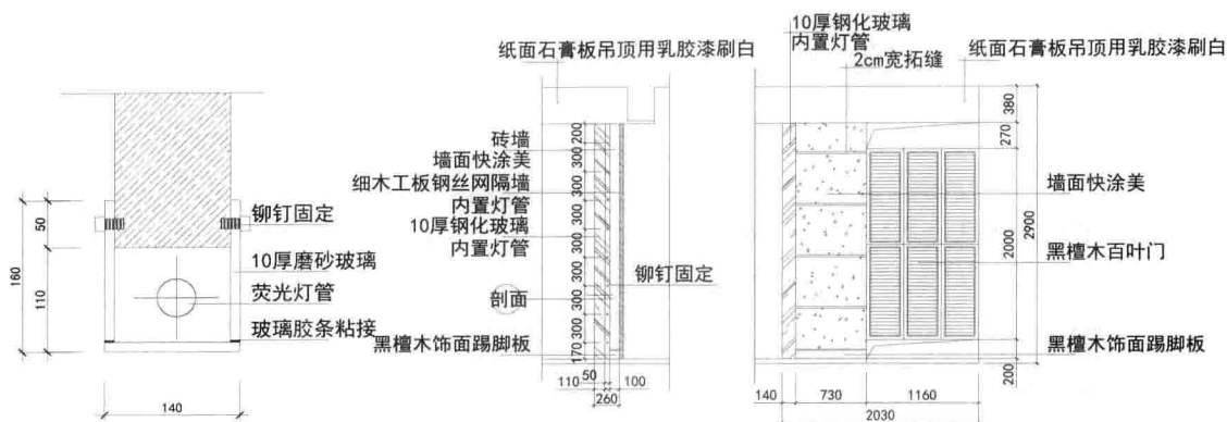
进门C立面图
