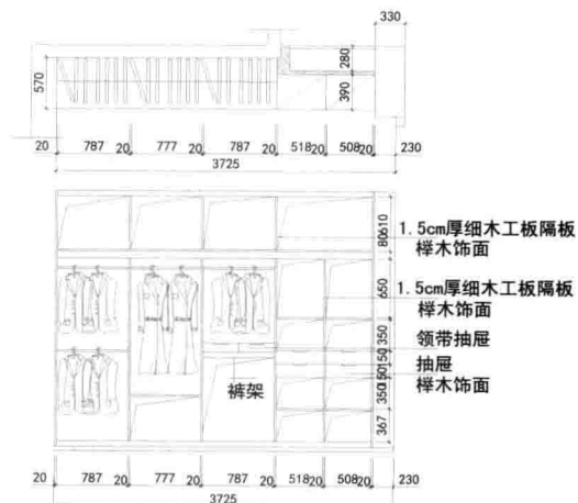
男孩房柜内部立面图
