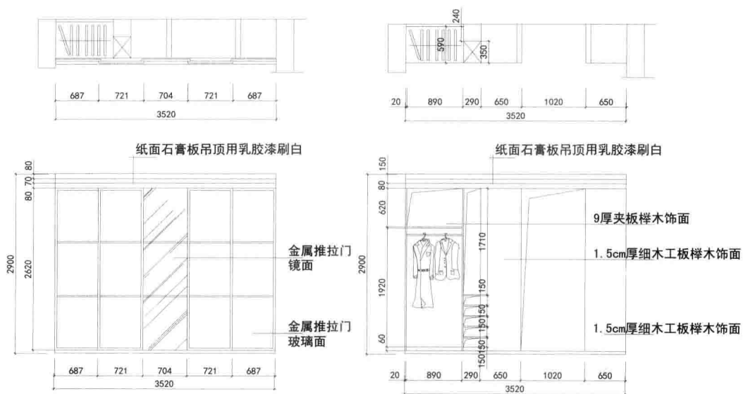
主卧室C立面图
