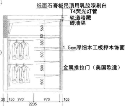
主卧室衣帽间 (内部) D立面图
