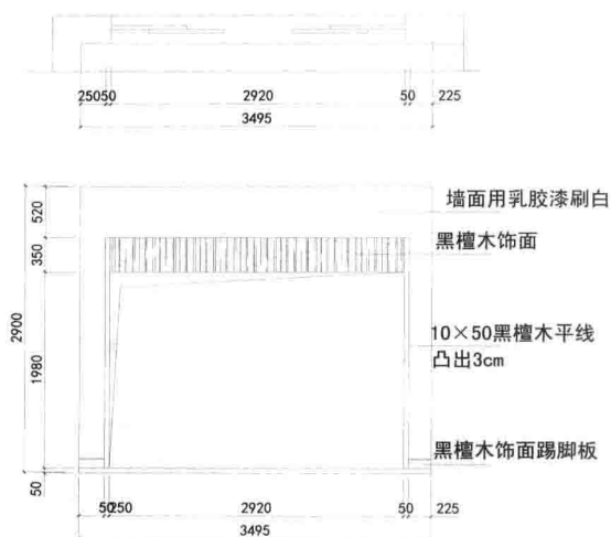
书房A立面图
