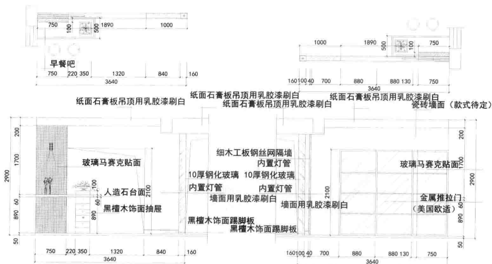
餐厅D立面图
