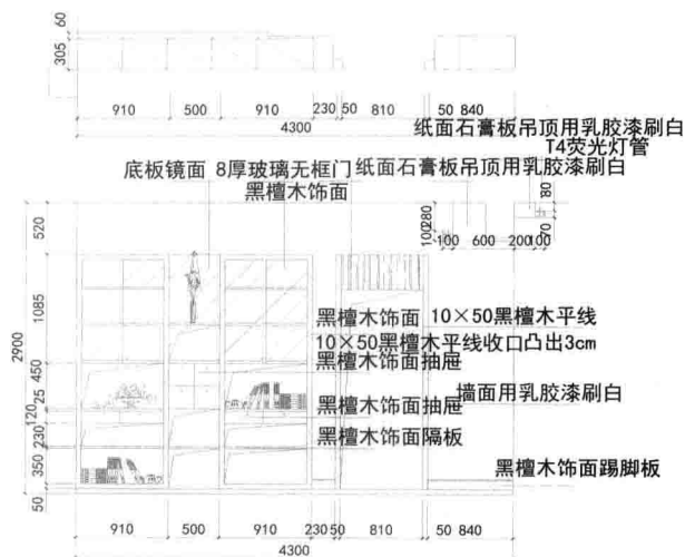
书房B立面图
