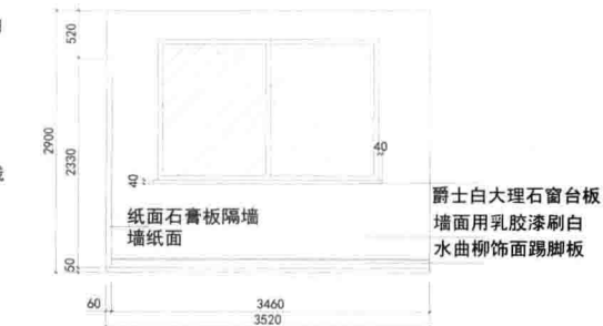
男孩房A立面图
