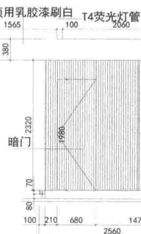
纸面石膏板吊顶用乳胶漆刷白 T4荧光灯管
