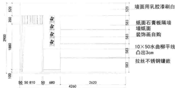
男孩房D立面图
