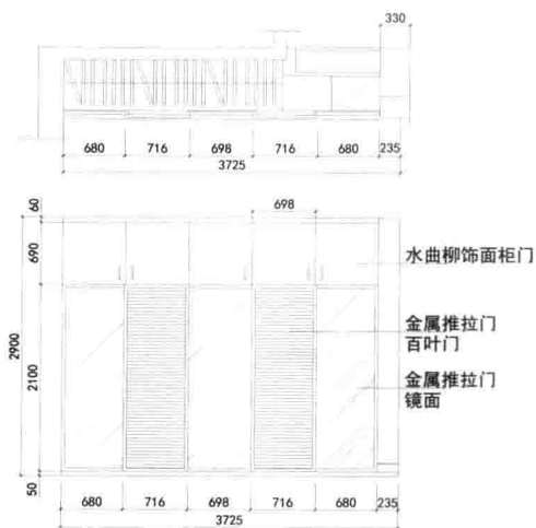
男孩房柜立面图
