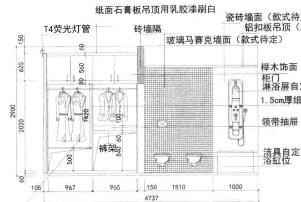
主卧室卫生间及衣帽间B立面图
