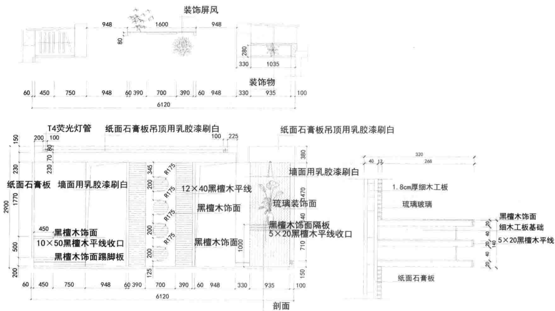
客厅A立面图
