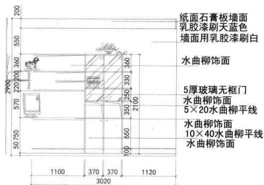
女孩房D立面图
