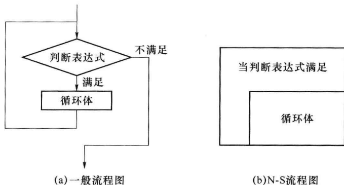
图 1-4 当型循环
