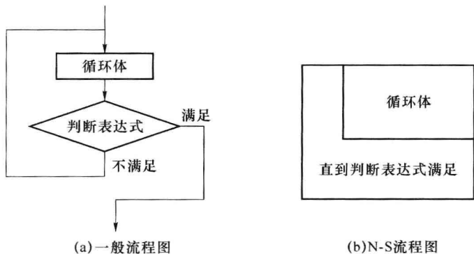
图 1-5 直到型循环
