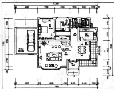
图 1-2 别墅施工图
