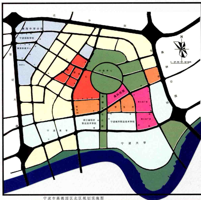
宁波市高教园区北区规划实施图
