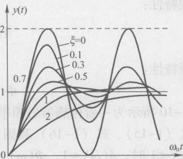
图 1-8 二阶传感器单位阶跃响应
