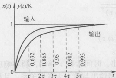
图 1-7 一阶传感器单位阶跃响应
