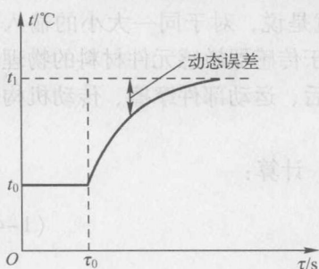
图 1-6 动态测温
