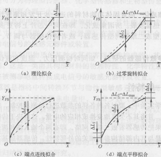
图 1-2 几种直线拟合方法
