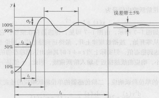
图 1-9 瞬态响应特性指标
