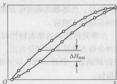
图1-4 迟滞特性
