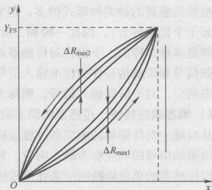
图1-5 重复性
