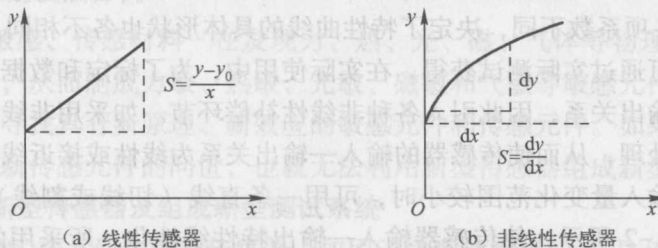
图 1-3 传感器的灵敏度
