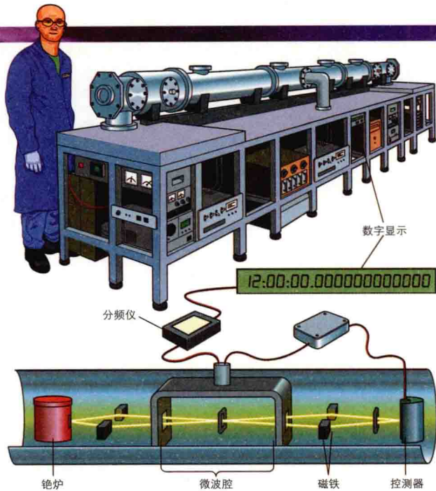
精确计时的铯原子钟（600万年才会误差1秒）
