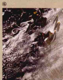
佛得角群岛影响了云层，出现了卡门涡街
