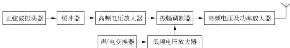
图 1-3 调幅无线电广播发射机的基本组成方框图
