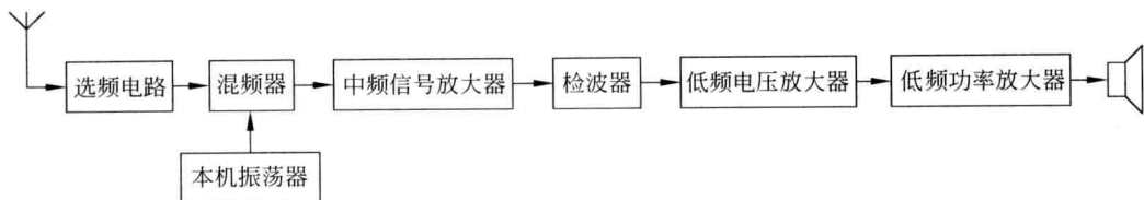
图 1-5 超外差式接收机的基本组成方框图
