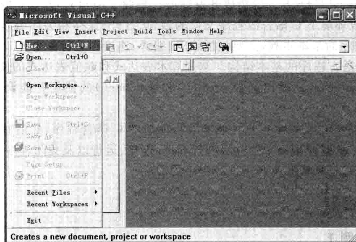
图 1-1-2 新建文件
