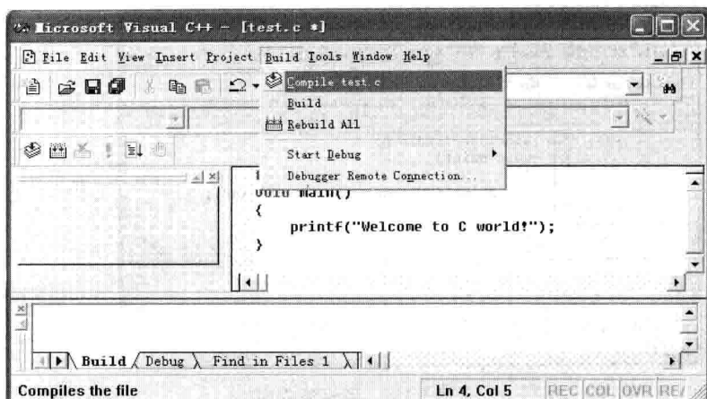
图 1-1-5 编译源程序
