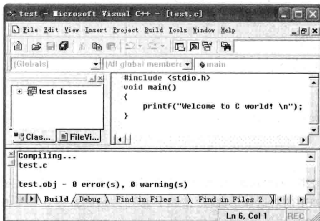
图 1-1-7 编译正确
