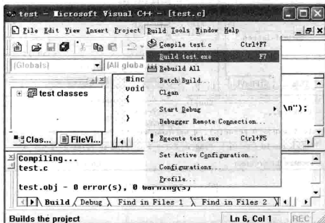
图 1-1-8 连接
