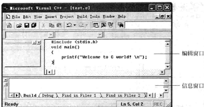
图 1-1-4 编辑源程序
