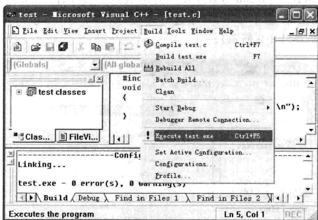
图 1-1-10 运行程序
