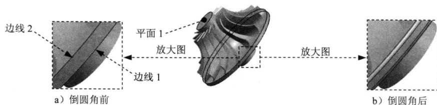
图 1.12 倒圆角 1
