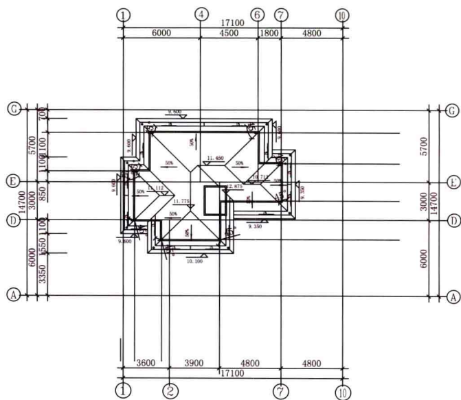
◆ 屋顶平面图
