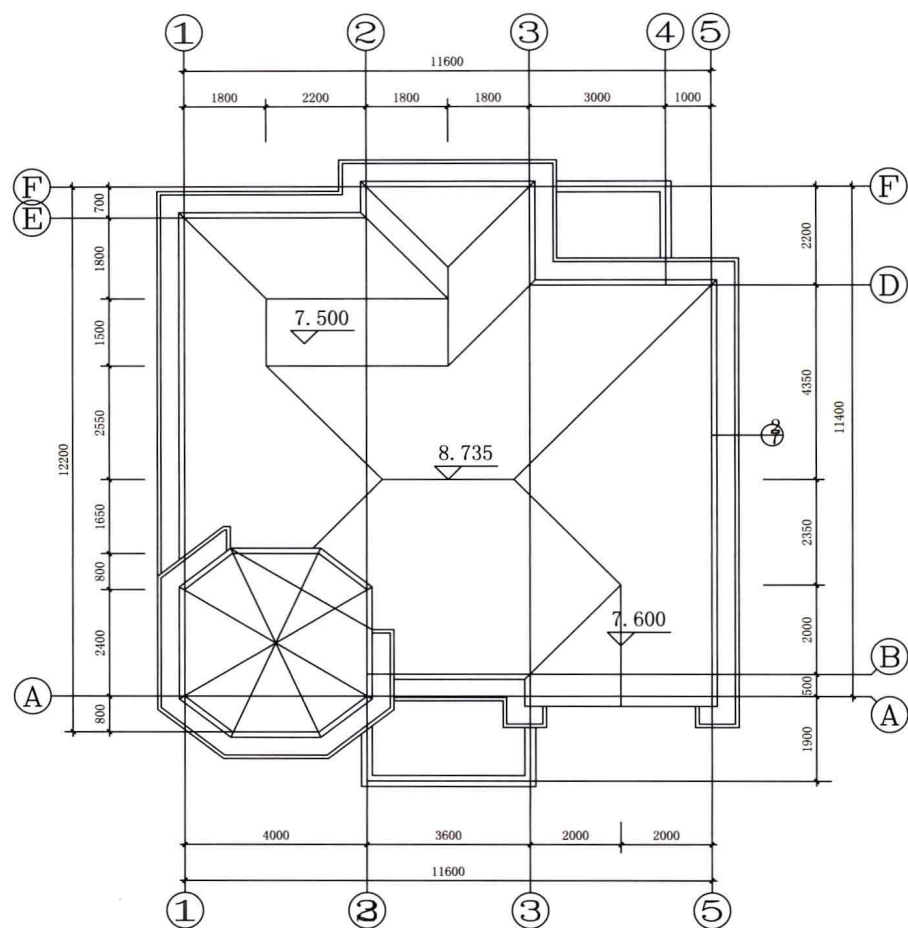
◆ 屋顶平面图
