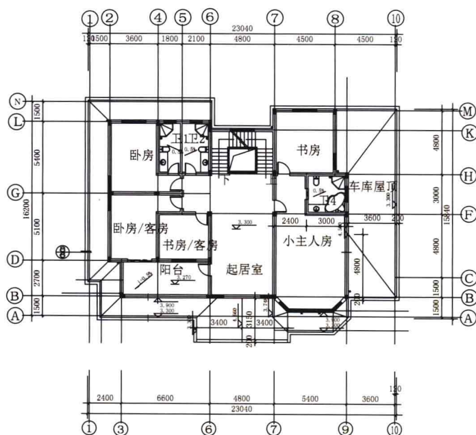
◆ 二层平面图
