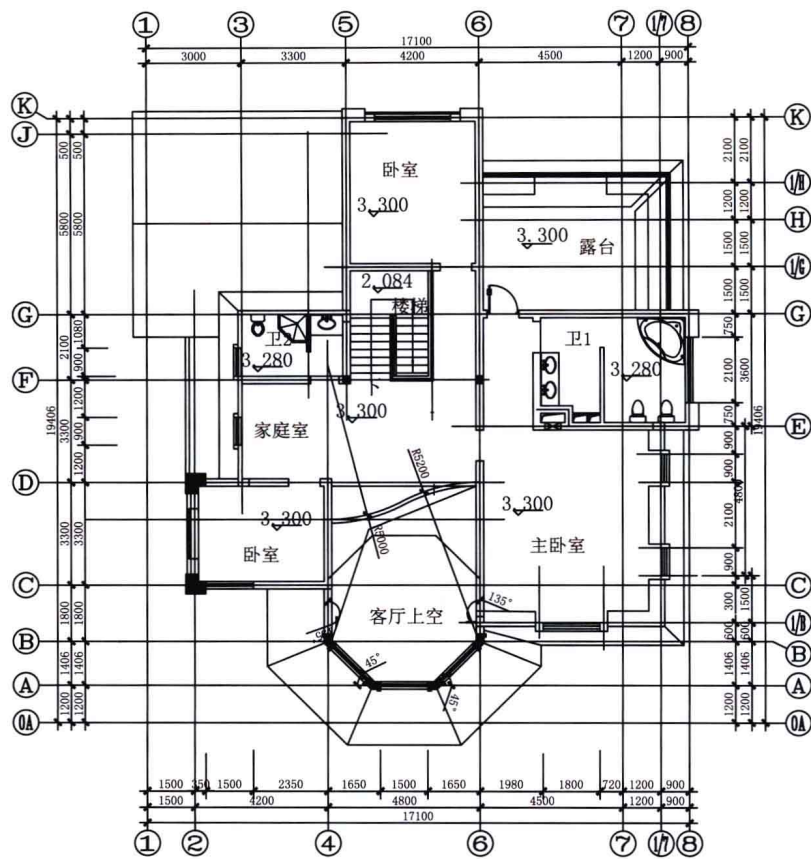
◆ 二层平面图
