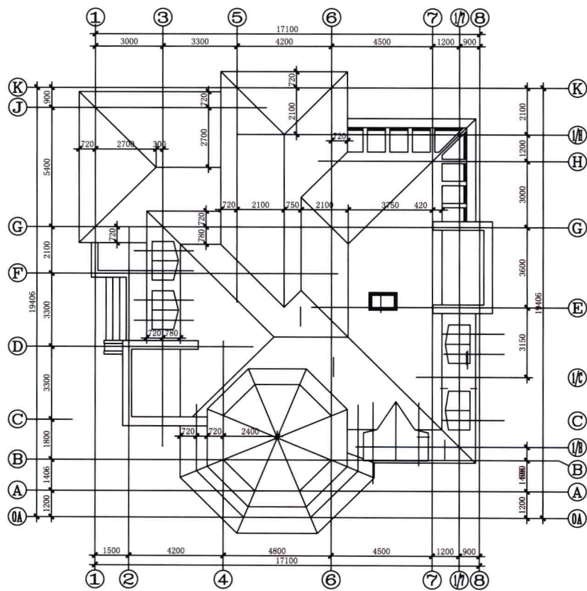
◆ 屋顶平面图
