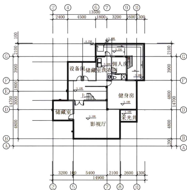
◆ 地下室平面图
