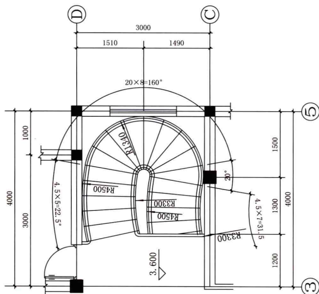
◆ 二层平面图
