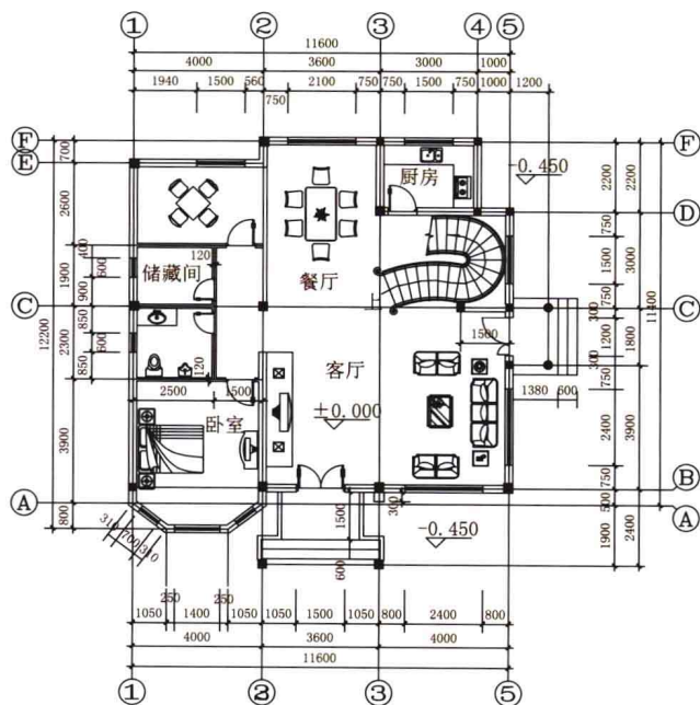
◆ 一层平面图
