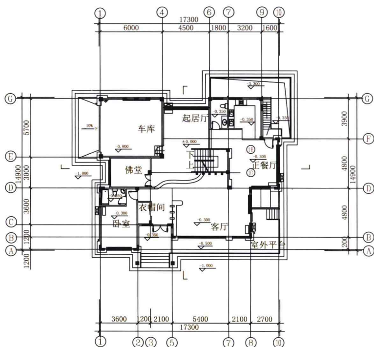
◆ 一层平面图
