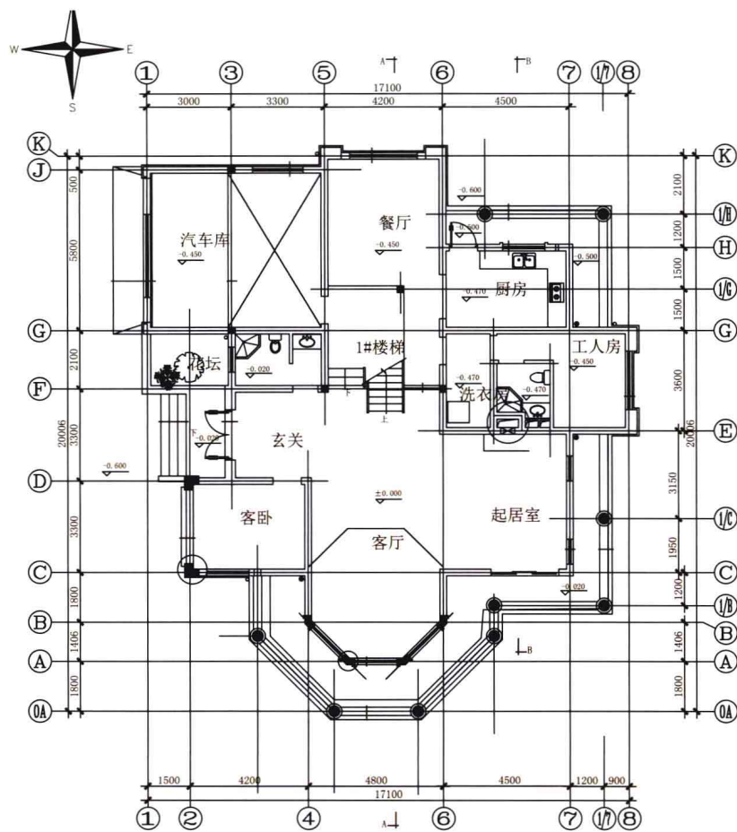
◆ 一层平面图
