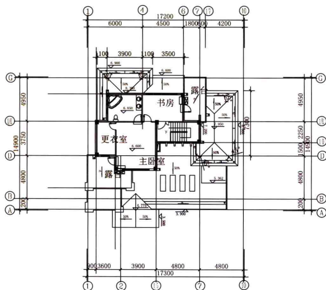
◆ 三层平面图
