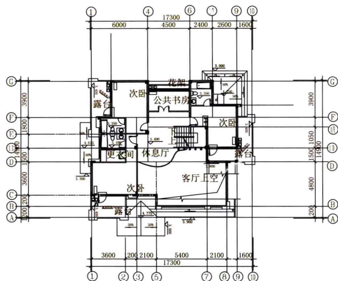
◆ 二层平面图
