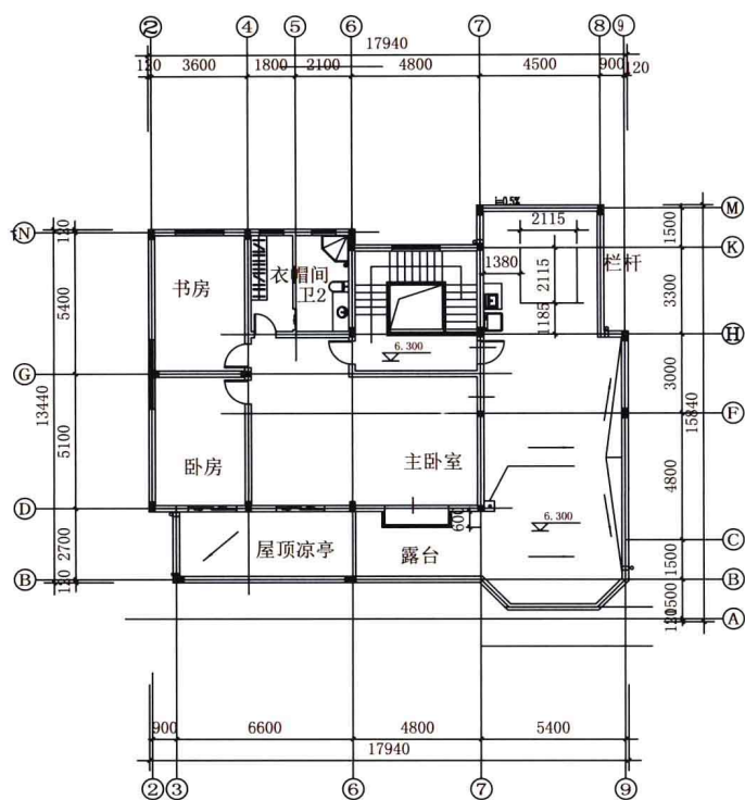
◆ 三层平面图
