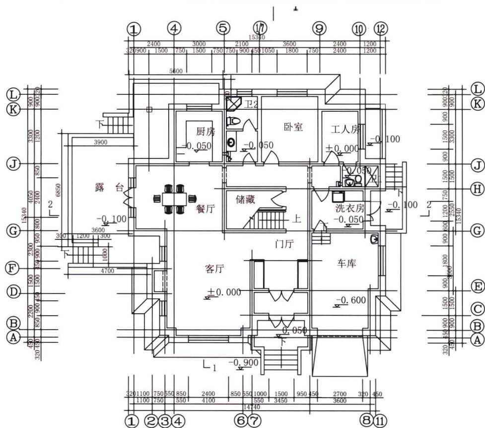
◆ 一层平面图
