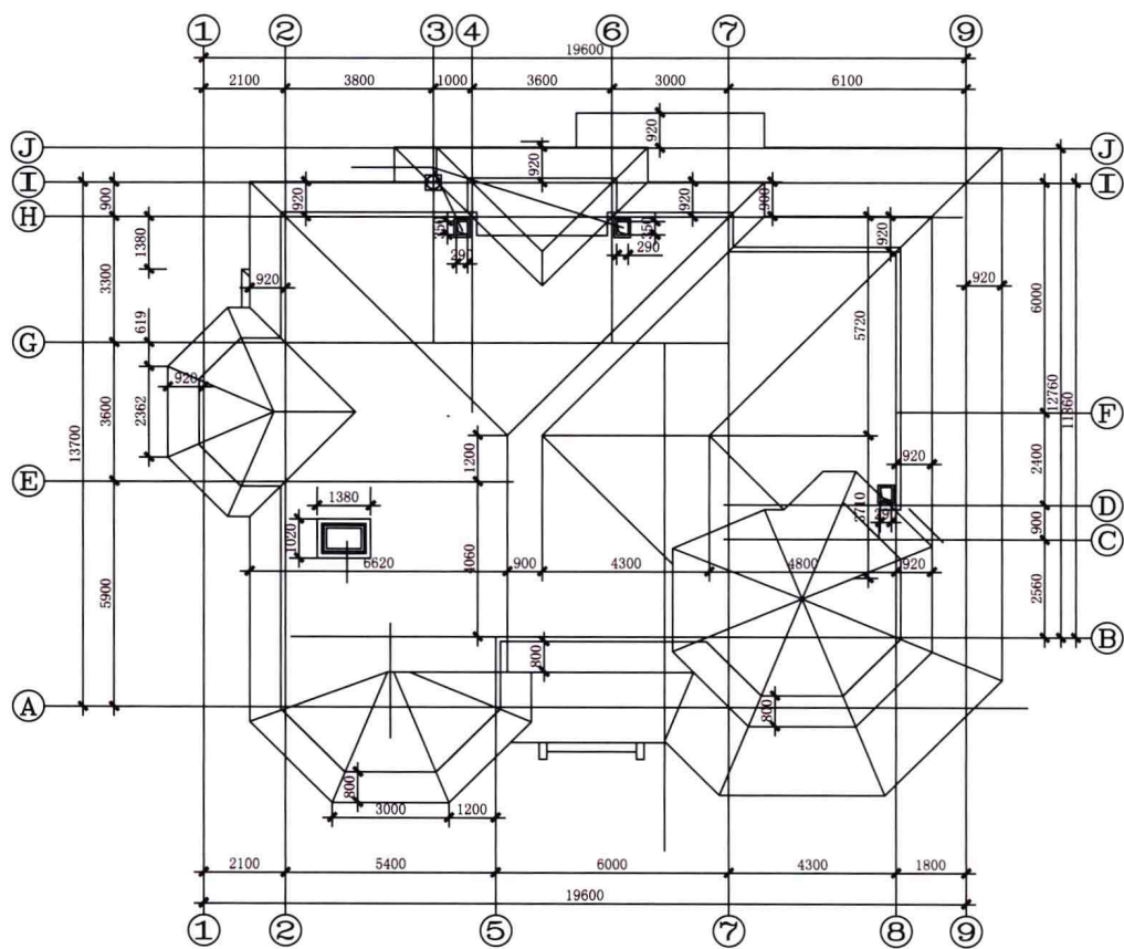
◆ 屋顶平面图
