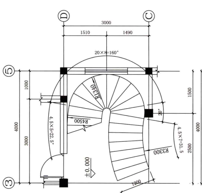
◆ 一层平面图
