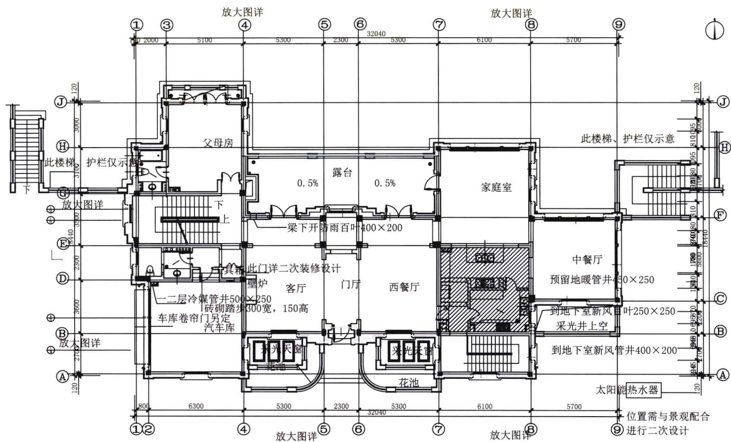
◆ 一层平面图
