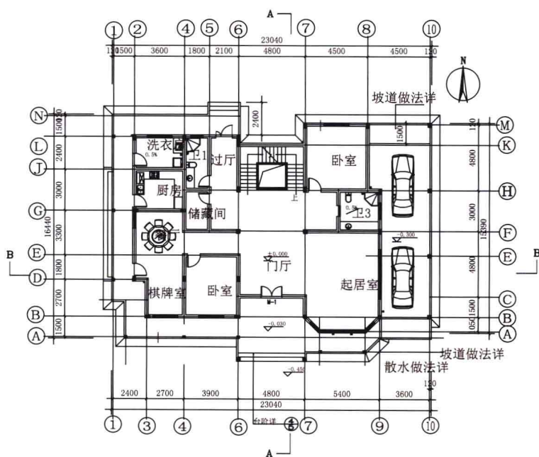
◆ 一层平面图
