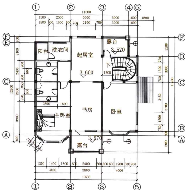
◆ 二层平面图
