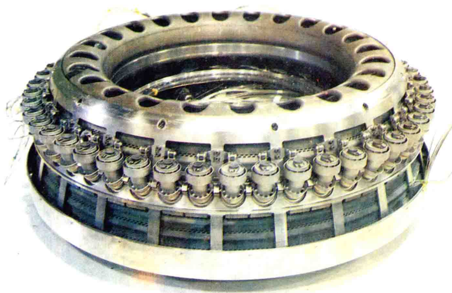
P & W 公司 高效节能 发动机双环腔燃烧室 总装图
