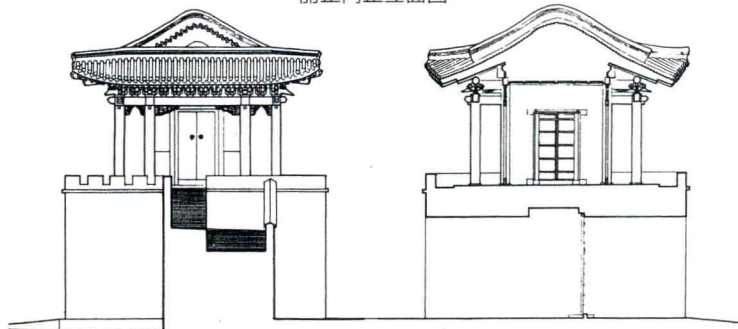
丽正门侧立面图
