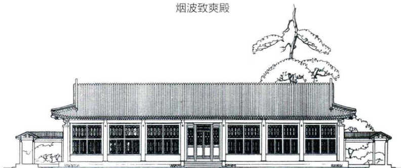
烟波致爽殿正立面图
