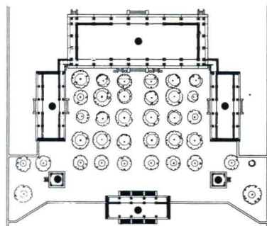
澹泊敬诚殿中庭平面图
