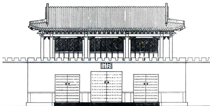
丽正门正立面图
