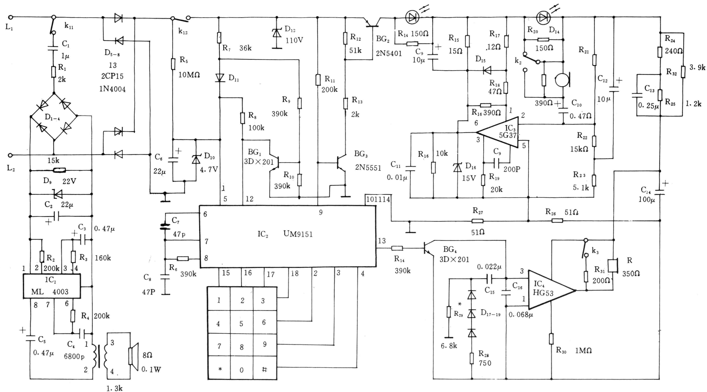
图1 HJ-1 型话机电路原理图
