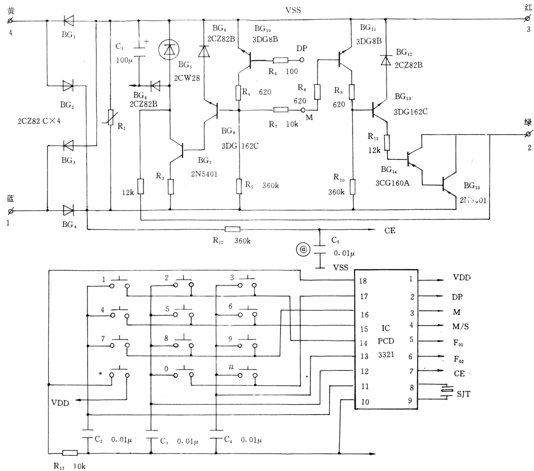
图 2 HZ-1P 型话机电路原理图
