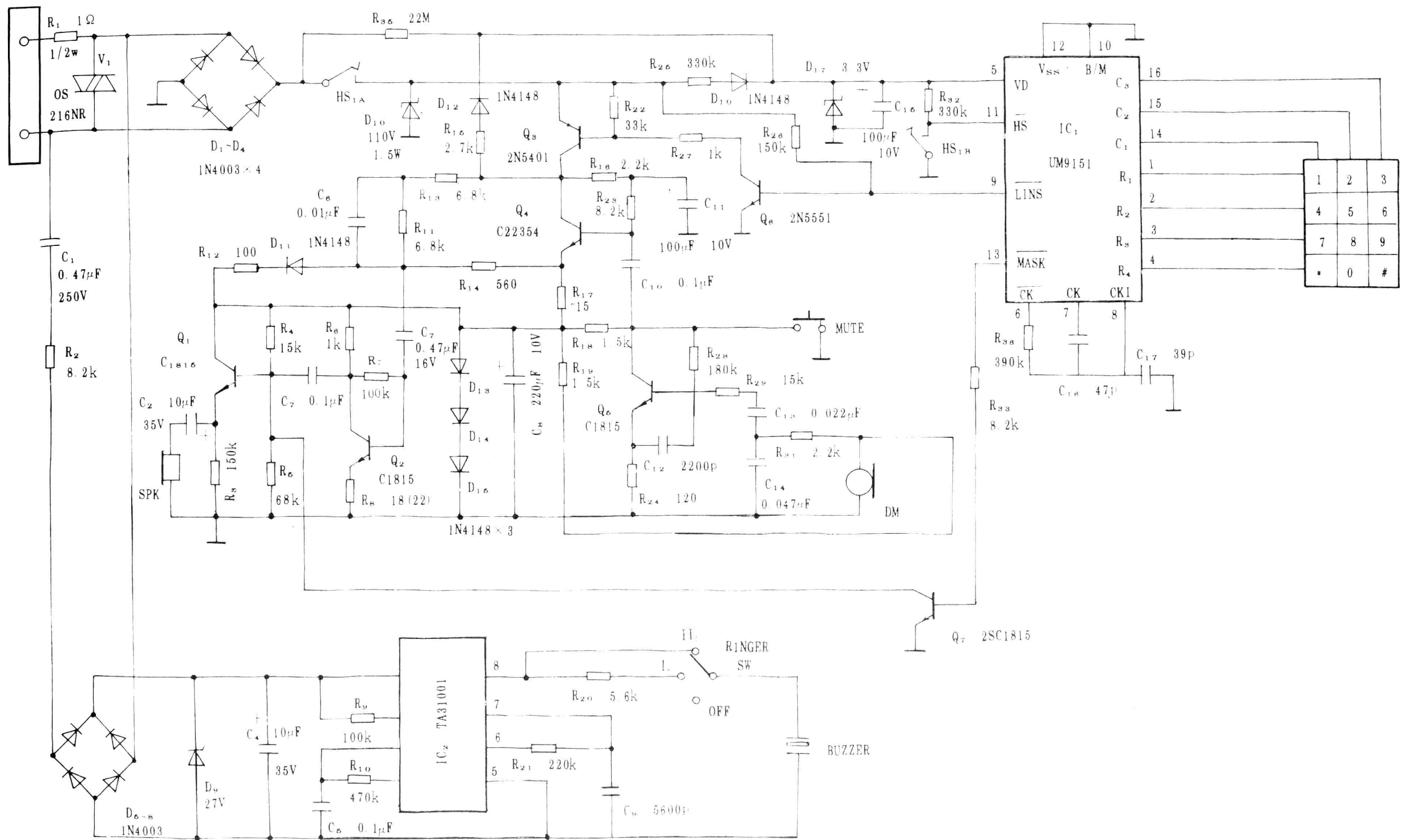
图 9 HA 011 型话机电路原理图
