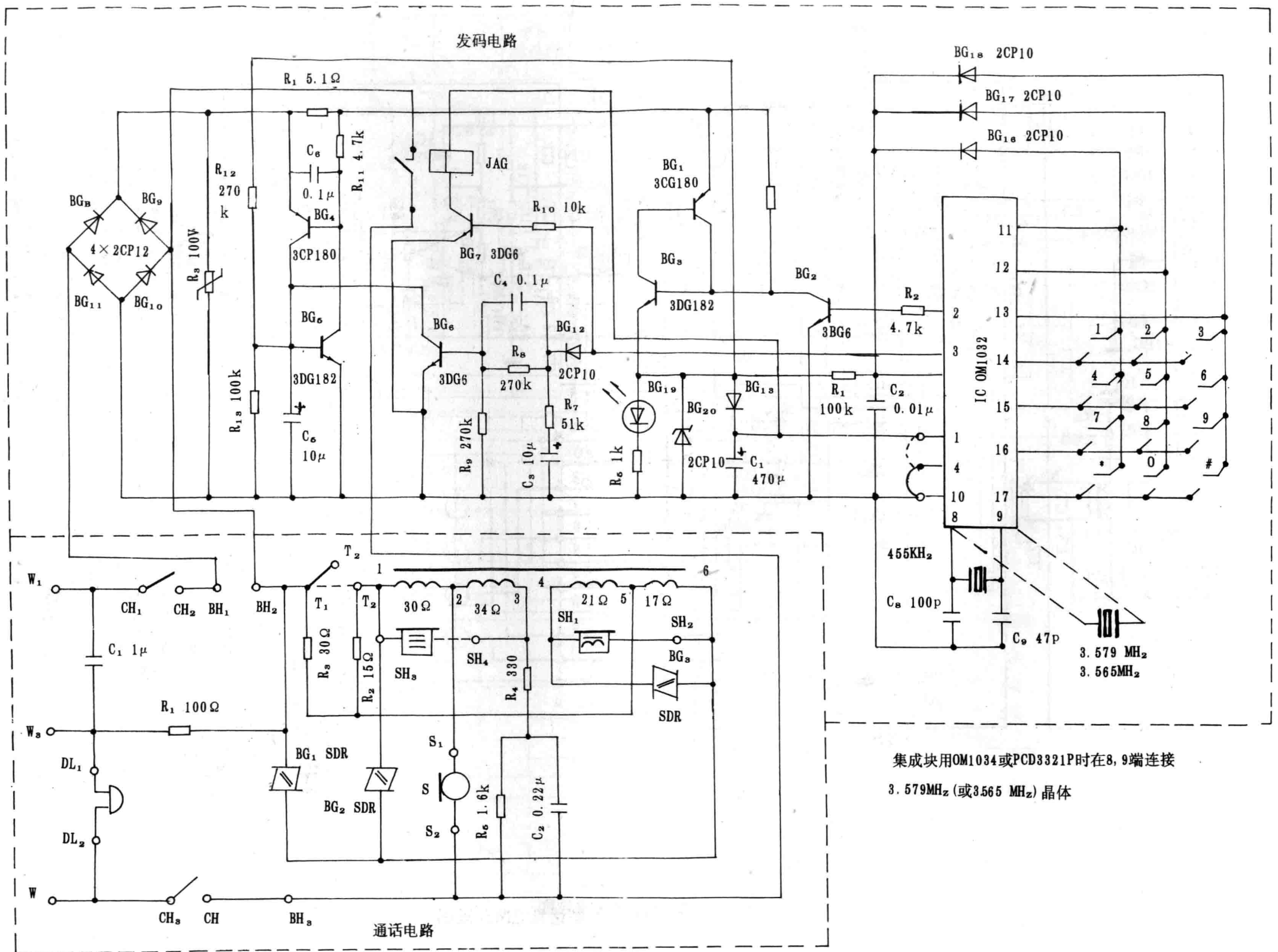
图4 HA-02型话机电路原理图
