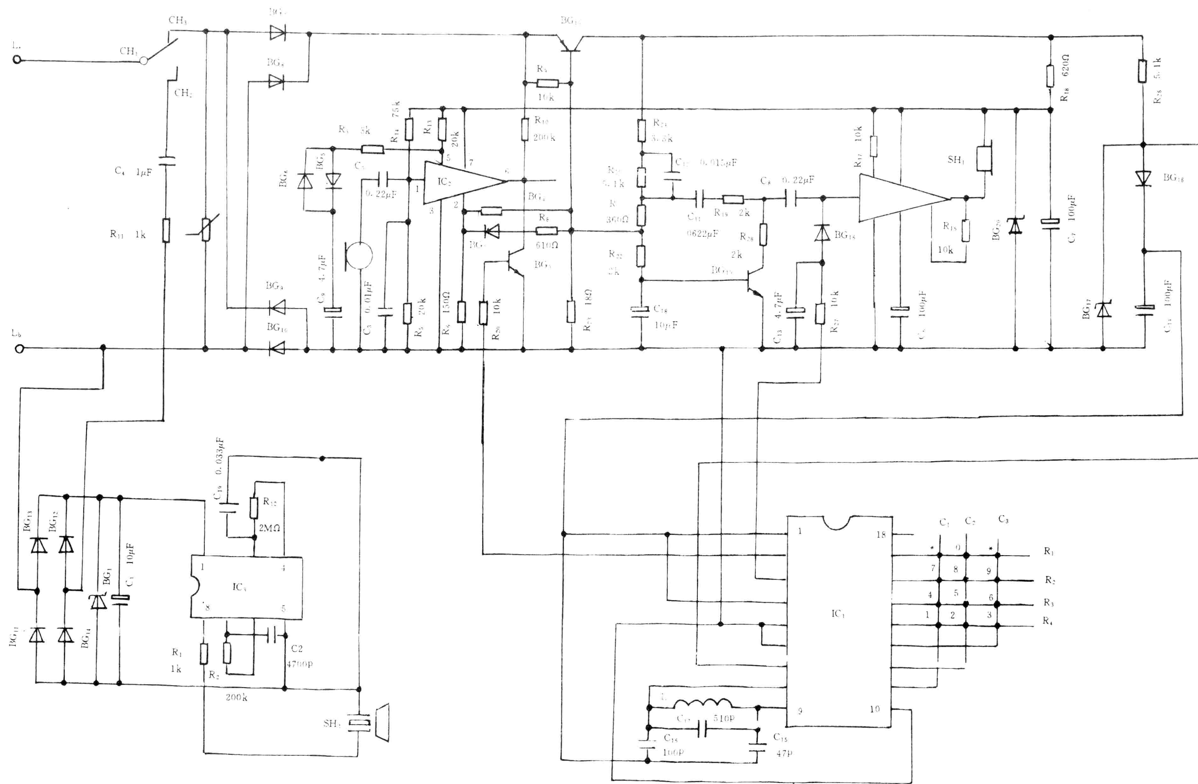
图 6 HA-04 型话机电路原理图
