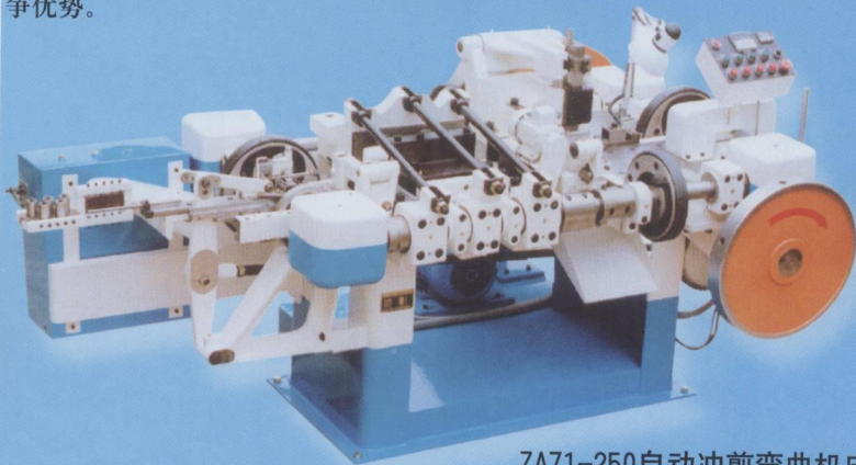
ZA71-250自动冲剪弯曲机床
