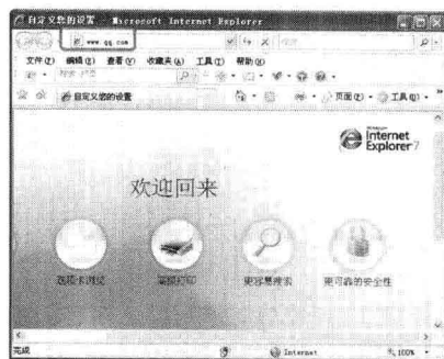
图 1-1 输入网址
