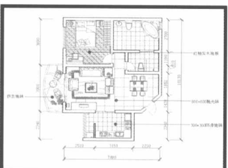
■ 尺寸及文字标注 (第20章) >>
