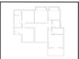
绘制阳台 (第13章) >>
