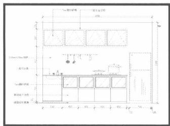
■ 标注尺寸和文字说明 (第18章) >>
