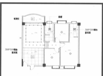
■ 跃层型天棚图 (第21章) >>
