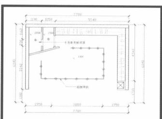
■ 服装店面天棚图模型 (第21章) >>
