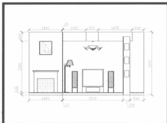
■ 标注尺寸 (第14章) >>
