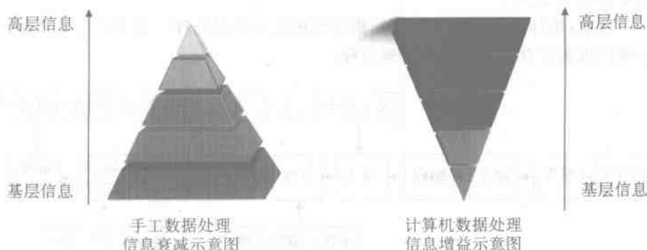
图 1.2.3 统计数据处理的信息增减示意图
