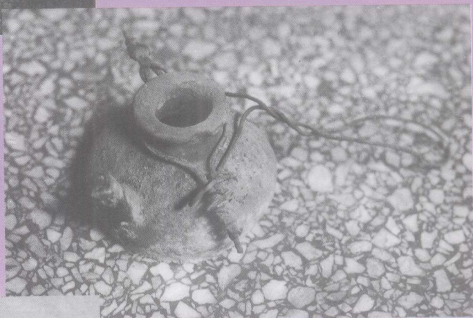
民国时期煤矿照明的亮油壶
