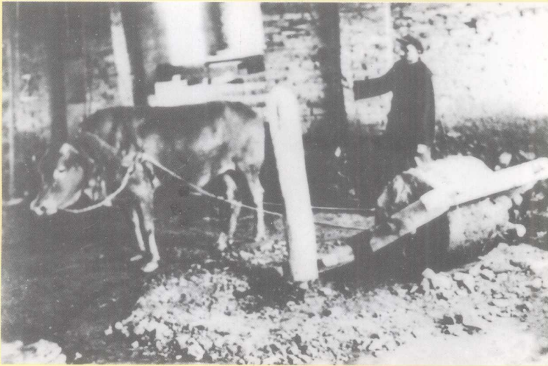
1964年永荣矿务局试制矸石砖牛拉碾碾碎矸石
