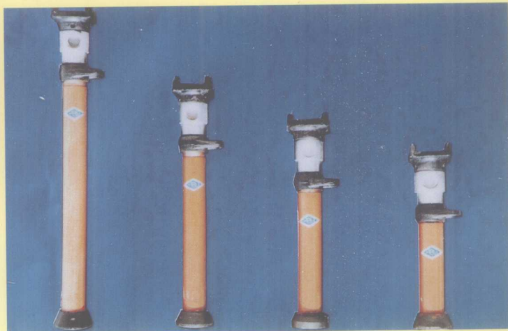
四川煤矿机械厂生产的单体液压支柱
