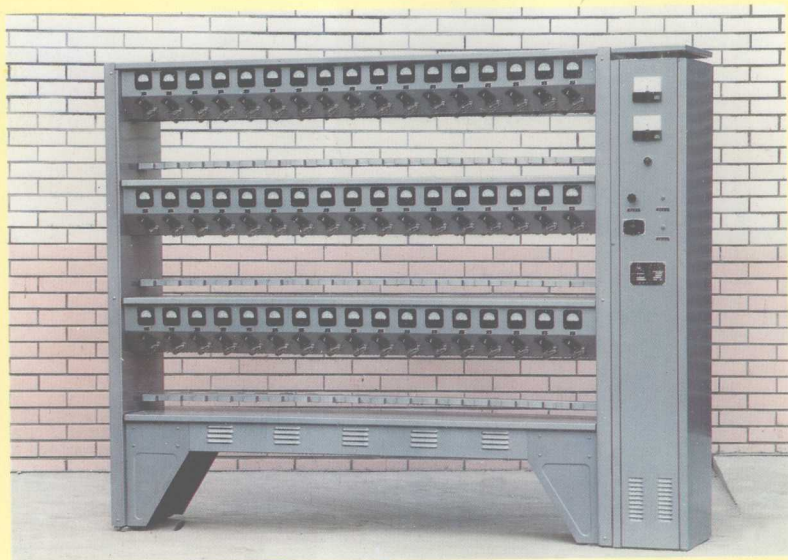
成都矿灯厂生产的矿灯充电架
