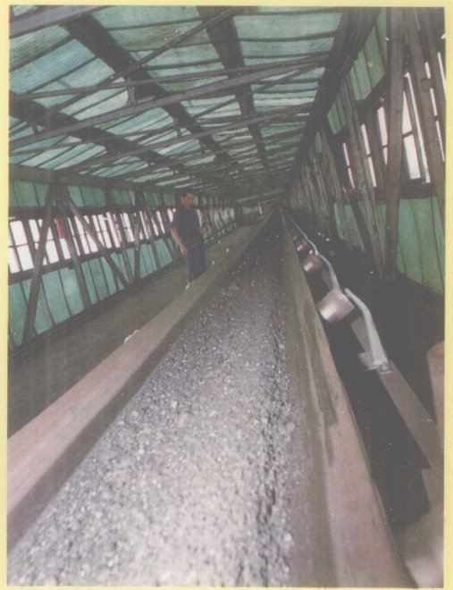
达竹矿务局渡市选煤厂胶带 走廊
