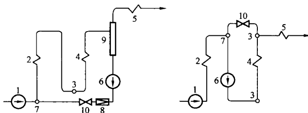
图 1-3 低倍率复合循环系统
