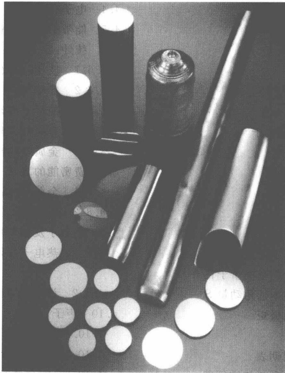
GaAs 晶锭和晶片
