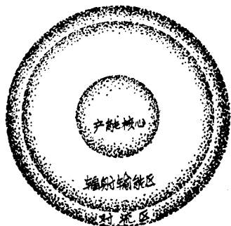
太阳内部结构示意图
