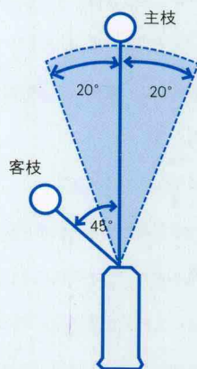
侧面图
