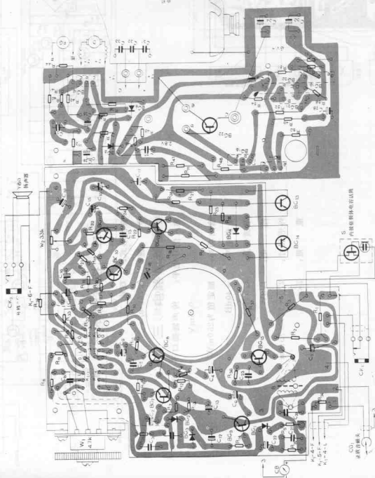
四、印刷电路板图
