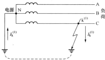
图 1-11 中性点直接接地系统电路图
