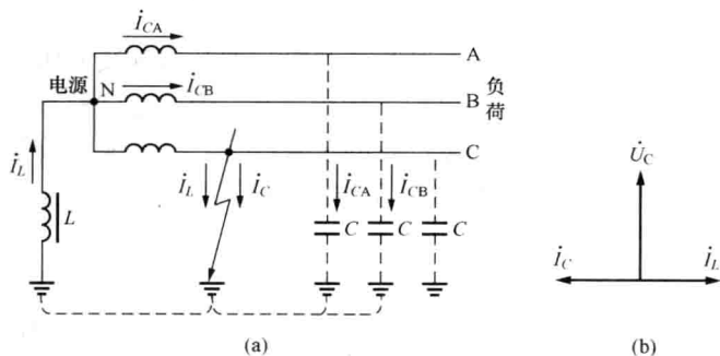
图 1-10 中性点经消弧线圈接地系统电路图
