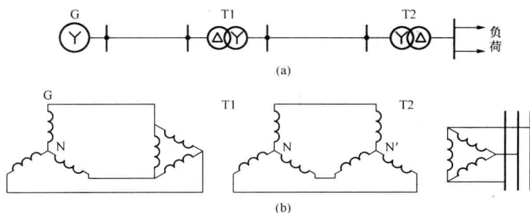
图 1-7 电力系统的中性点示意图
