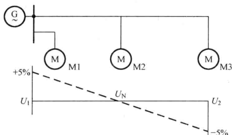
图 1-5 用电设备和发电机的额定电压
