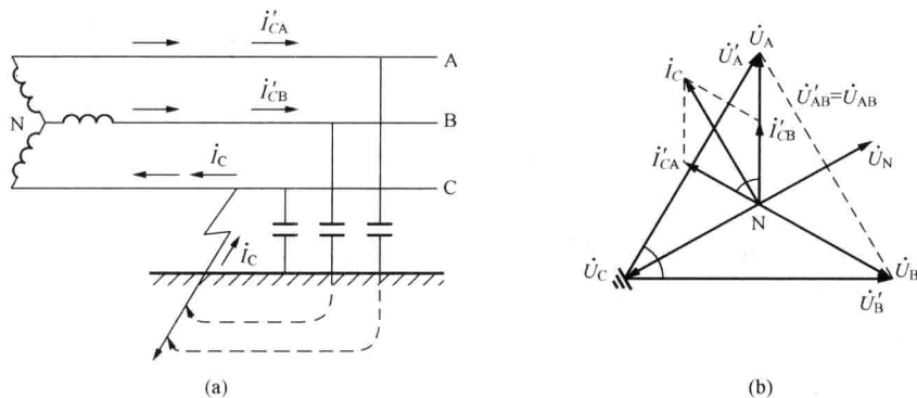
图 1-9 中性点不接地系统 C 相接地的情况
