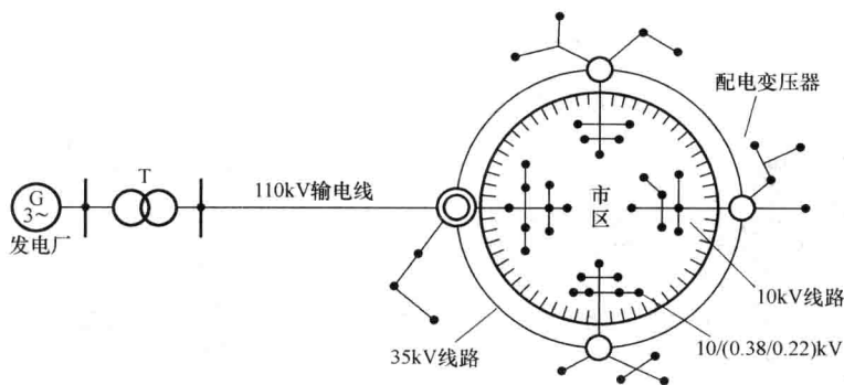
图 1-3 城区供电网电能的输送和分配示意图
