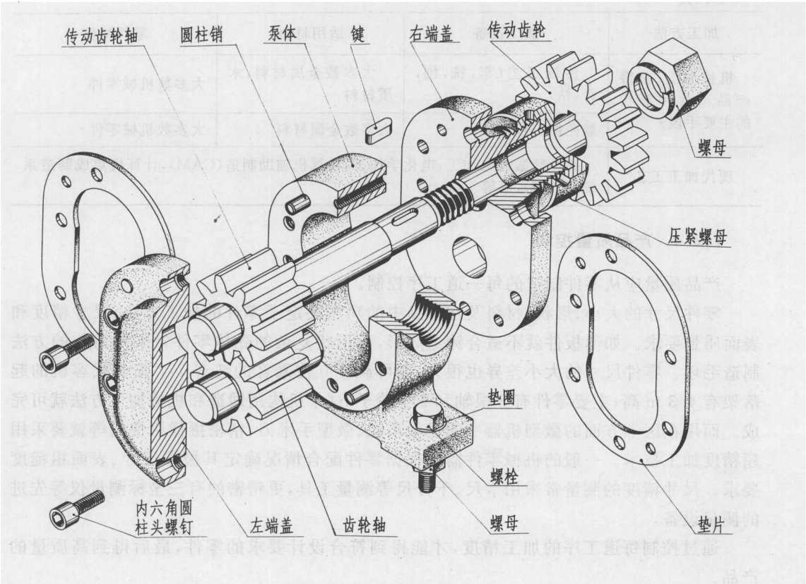
图 1-3 齿轮油泵分解轴测图
