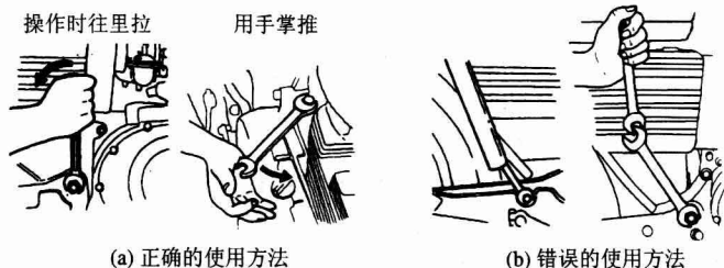
图 1-4 开口扳手的使用
