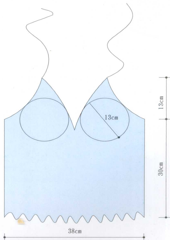
前片结构图
