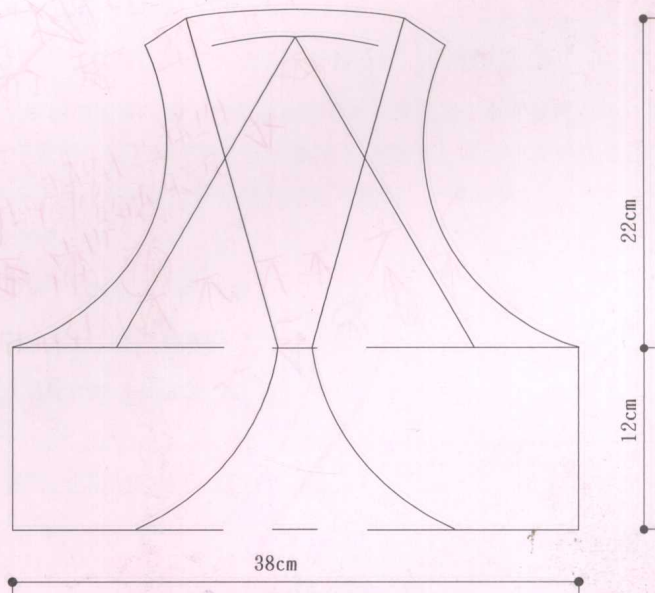
后片结构图
