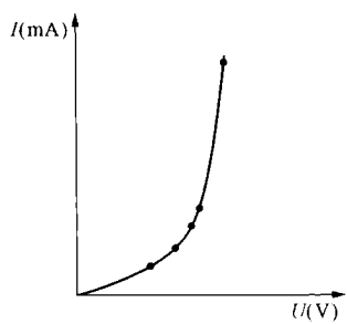
图 1-1 PN 结正向特性曲线
