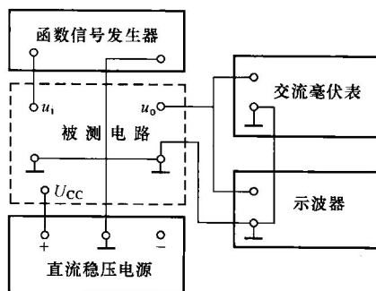
图 2-1 电子电路中电子仪器与被测实验装置之间的布局与连接
