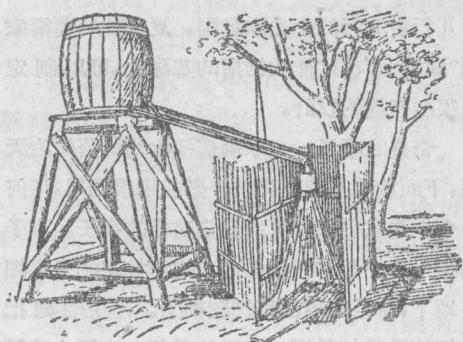
夏令营中的自制淋浴器
