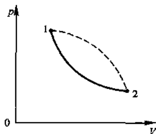
图 1-8 准静态过程和非准静态过程
