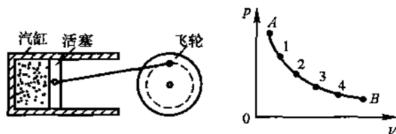
图 1-9 可逆过程图
