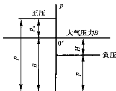
图 1-6 各压力间的关系
