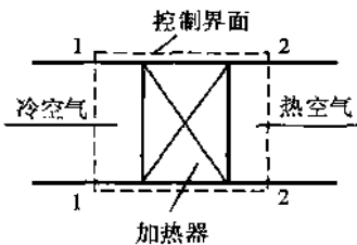
图 1-3 开口系统
