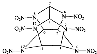
图 1-1 HNIW 的结构图
