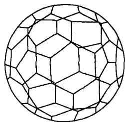
图 1-6 富勒烯
