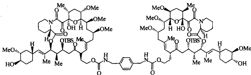
图 1-5 FK-1012
