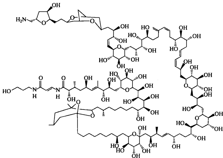
图 1-3 海葵毒素
