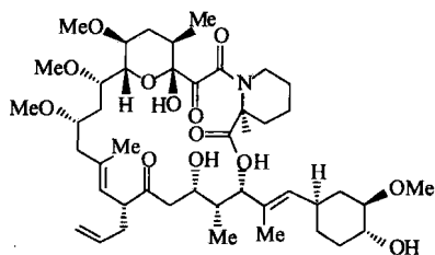
图 1-4 FK-506
